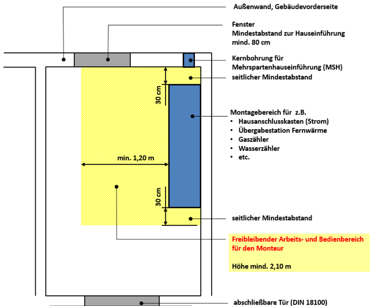
Abb. Beispiel Hausanschlussraum
