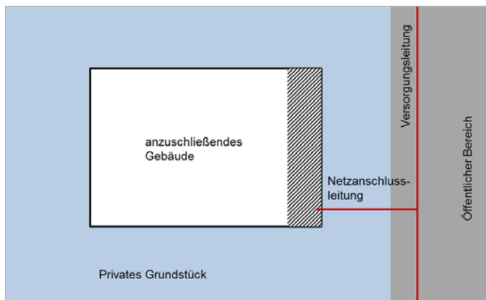
Abbildung 3 Anordnung des Übergabeschachts
