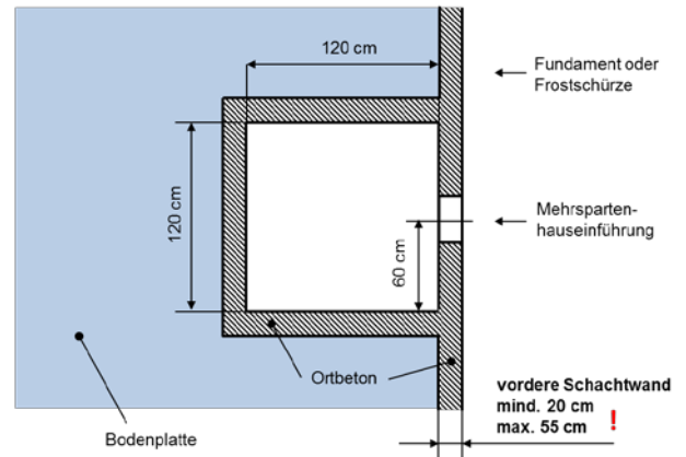
Abbildung 2 Übergabeschacht: Draufsicht
