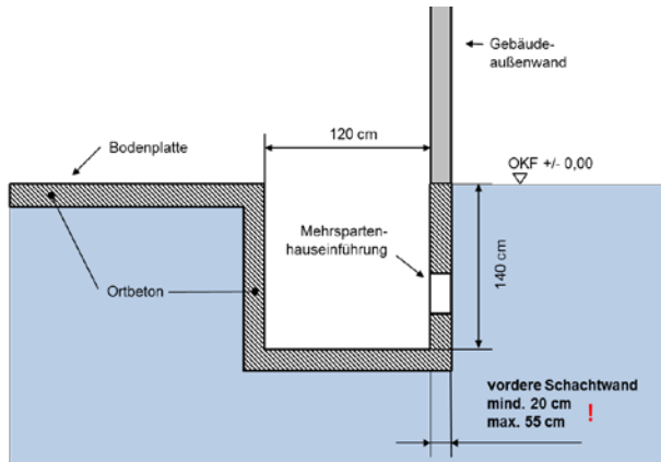
Abbildung 1 Übergabeschacht: Schnittzeichnung
