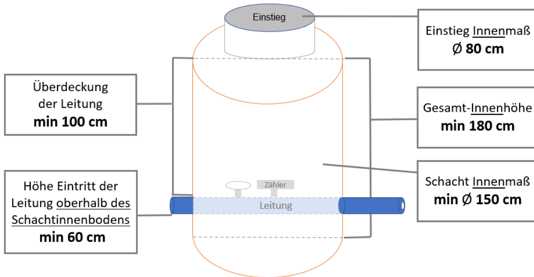
Abb. 4: Runder Betonschacht als Übergabe- und Zäblerschacht
