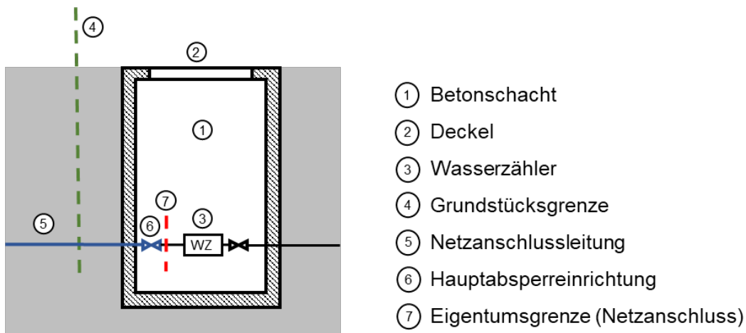
Abb. 2: Schematische Darstellung der Anordnung eines Betonschachts
