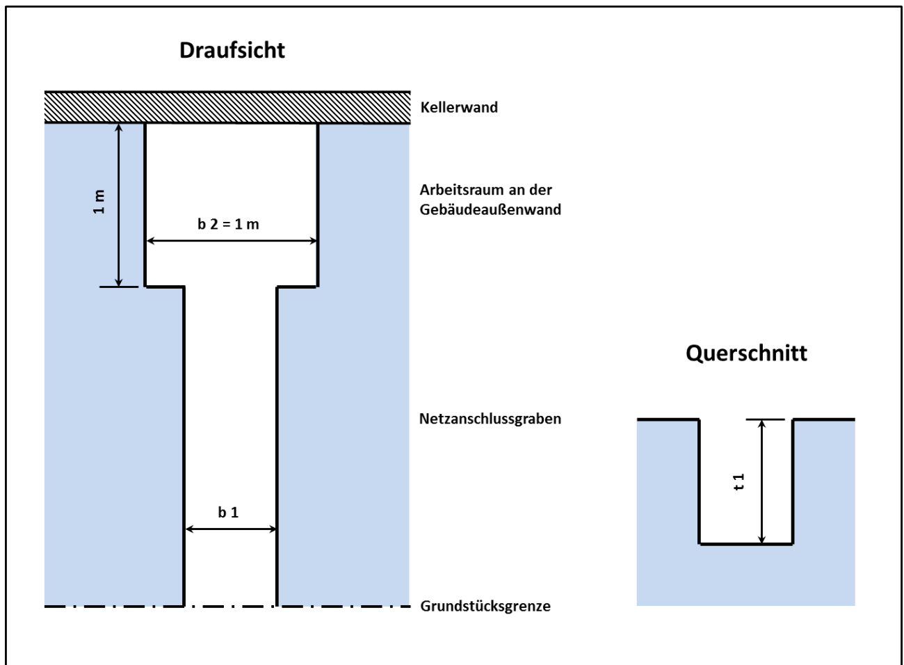
Abbildung 1: Grabenprofile und Maße
